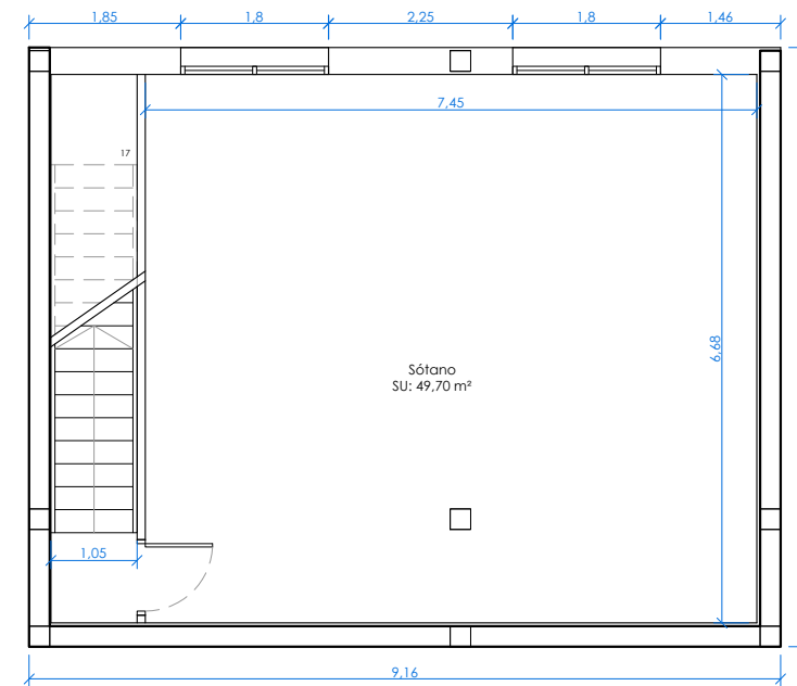
OPCIÓN SÓTANO
