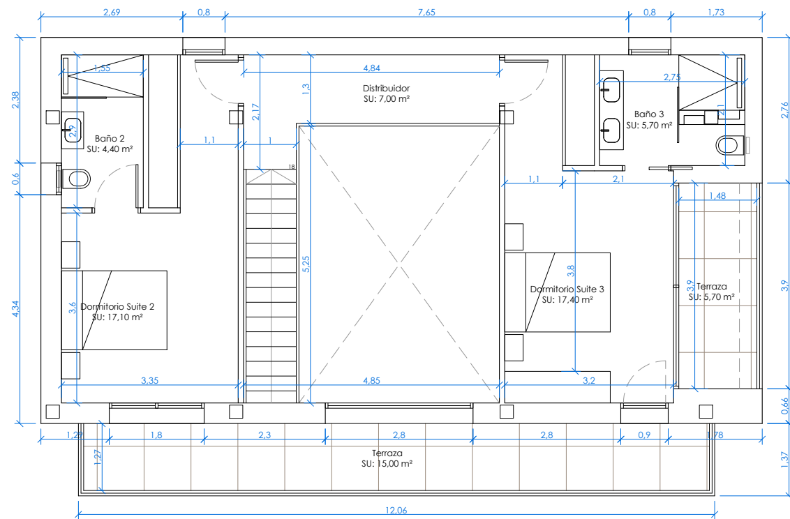
PLANTA PRIMERA
