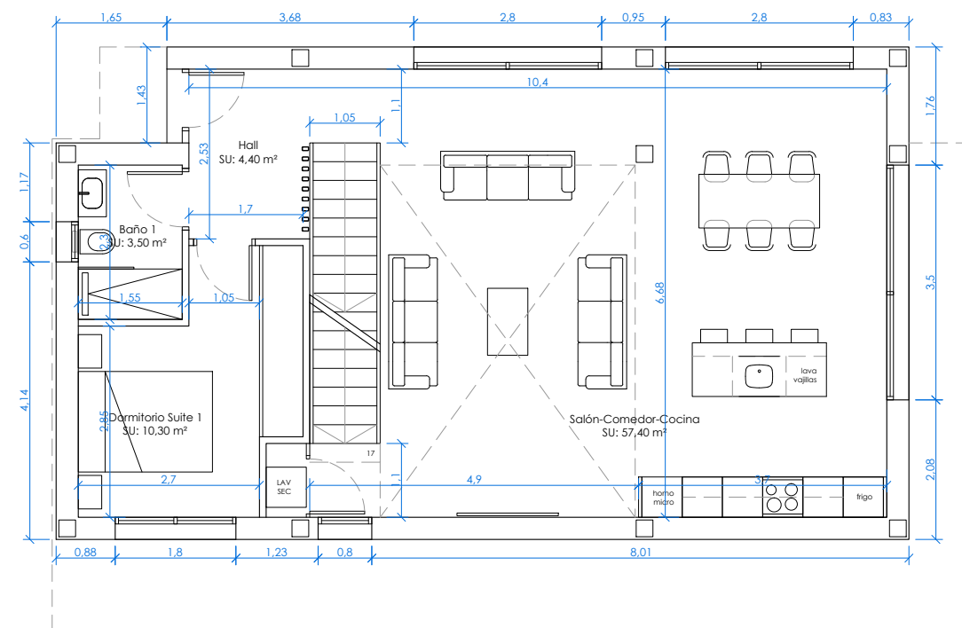
PLANTA BAJA
