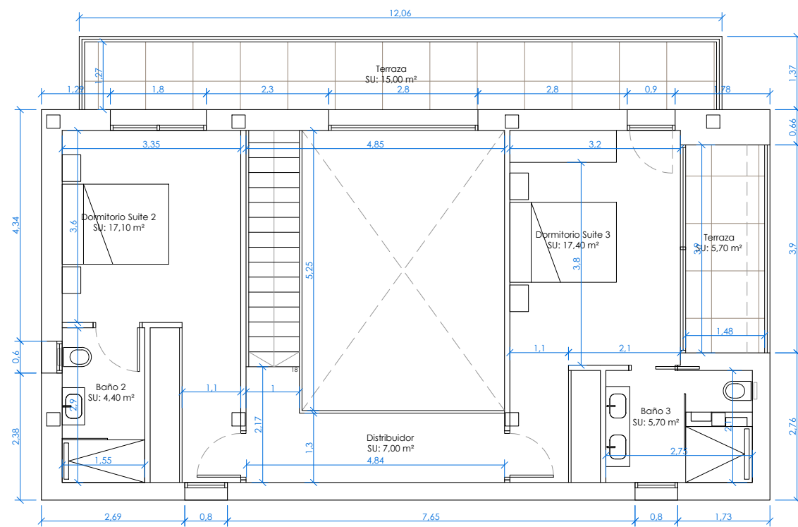
PLANTA PRIMERA
